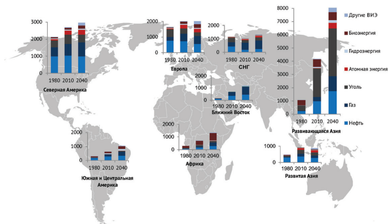
Рис. 1.22. Потребление первичной энергии по регионам и видам топлива, Базовый сценарий, млн т н.э.
