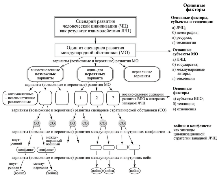
Рис. 1.24 116 . Логика анализа и долгосрочного прогноза международной обстановки, будущего характера международных и внутренних войн и военных конфликтов
