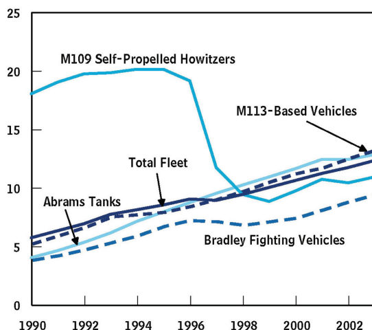
Рис. 1.14. Средний возраст (в годах) боевых средств Армии США (Average Age of the Army's Armored Combat Vehicles, 1990 to 2003)
